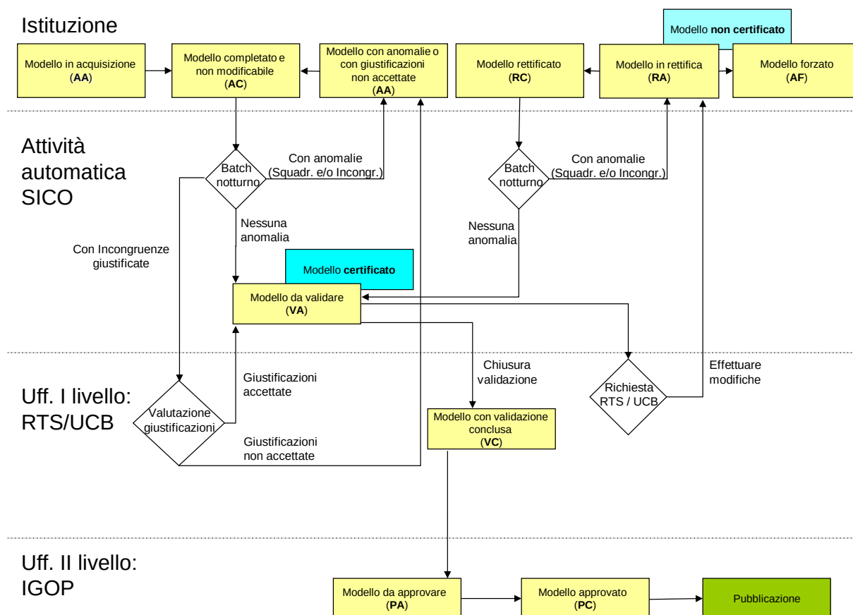
Figura 1 – Il processo di lavorazione dei dati in SICO
